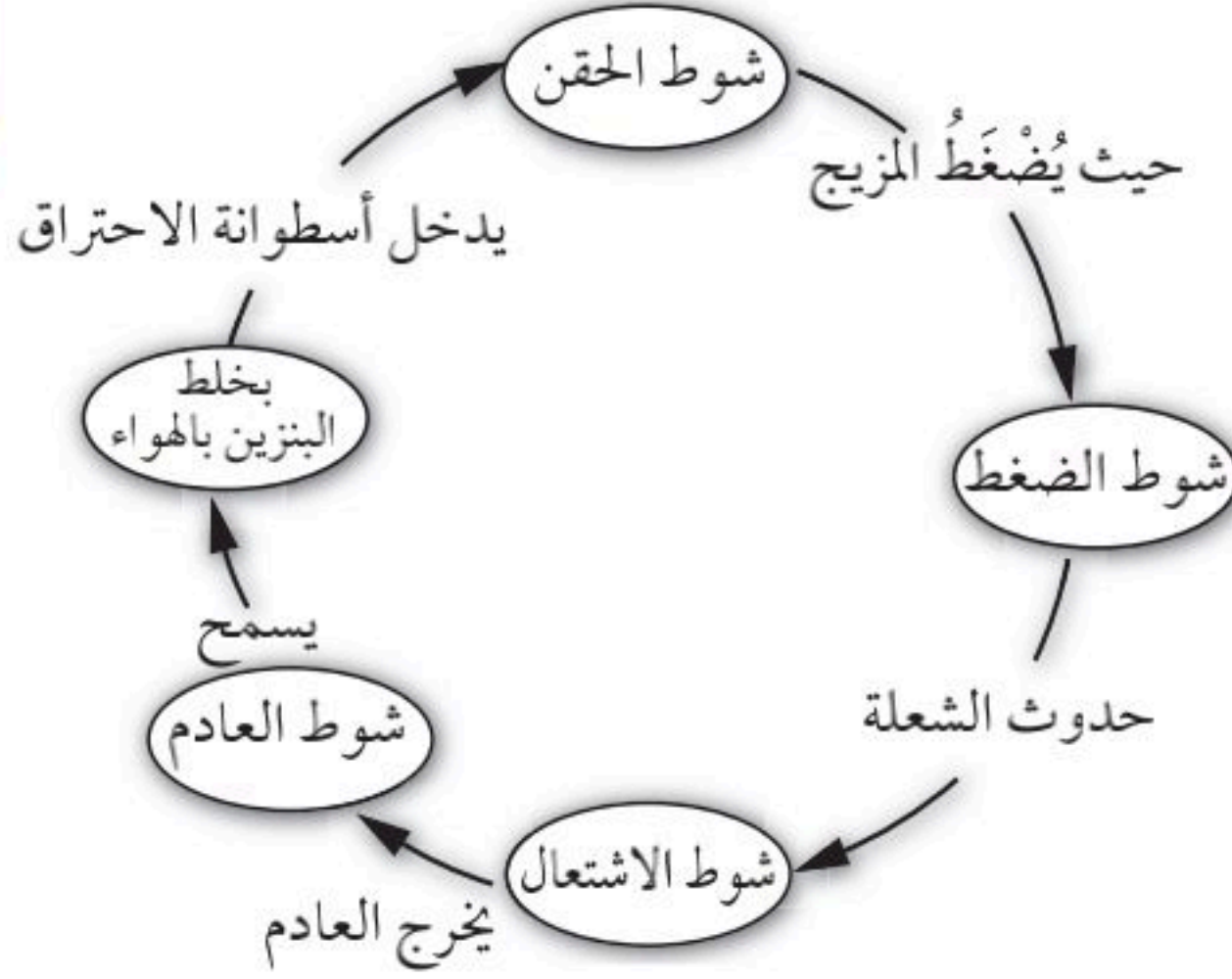
الشكل ٤ تظهر خريطة الدورة الأحداث التي تحدث في آلة الاحتراق الداخلي.
