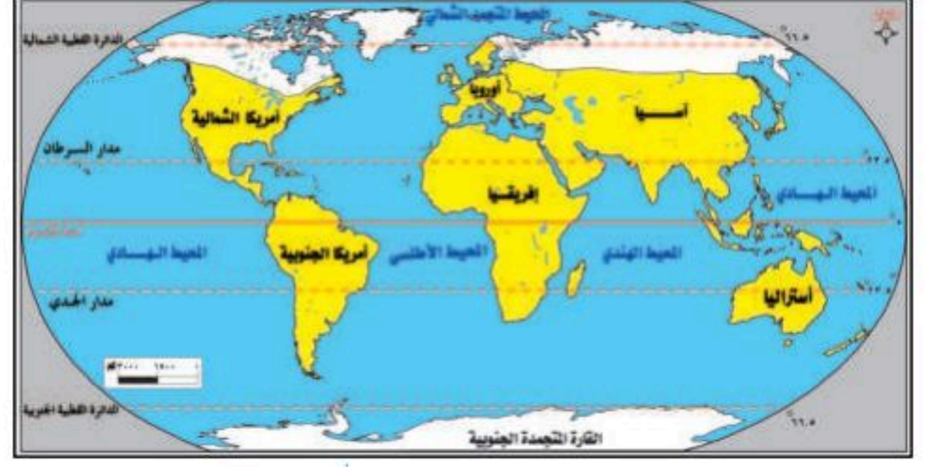
الشكل ٢٥ تتكون الجليديات في المناطق الباردة
