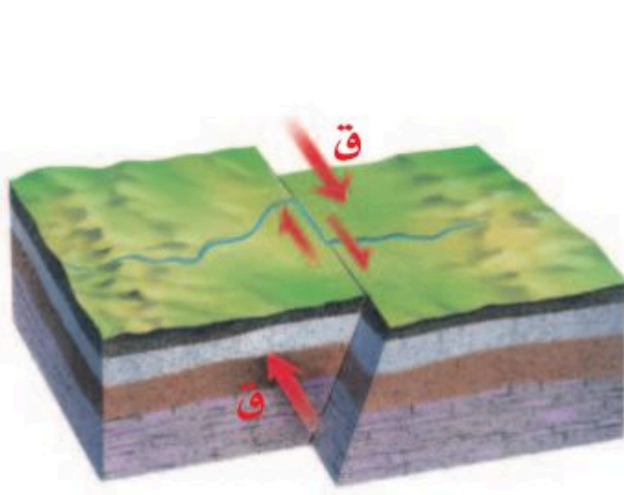
ج ينتج الصدع الجانبي (الانزلاقي) عندما تتعرض الصخور لإجهادات قص (تؤثر فيها بصورة جانبية).
