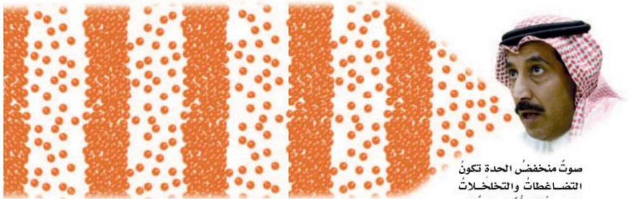
صوت مرتفع الحدة تكون التضاعطات والتخلخلات متقاربة (تردد عالٍ)
